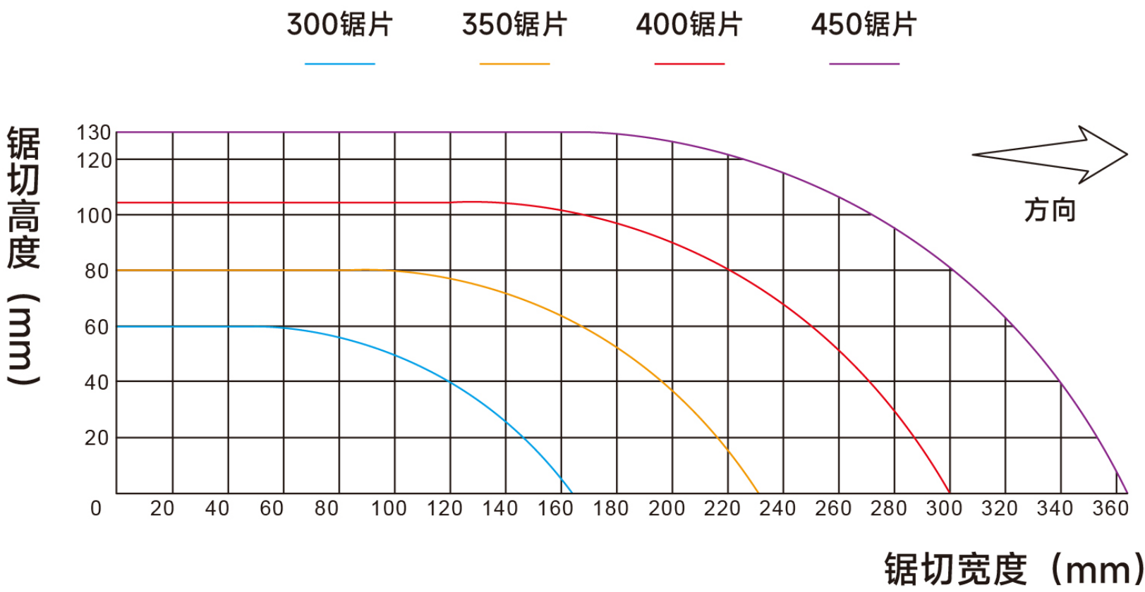
锯切能力图（横向）
